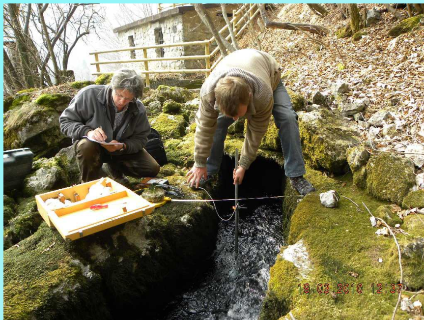
Misure di portata con mulinello idrometrico
